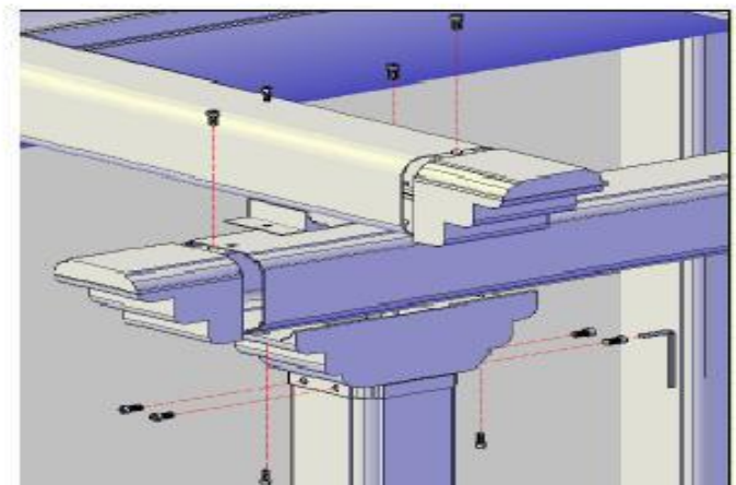
MONTAJE PARTE SUPERIOR
