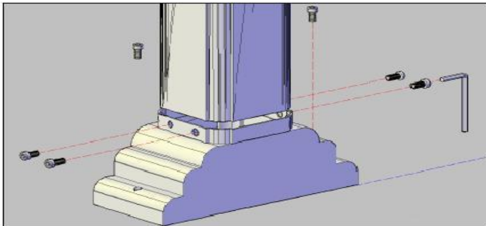
MONTAJE PARTE INFERIOR
